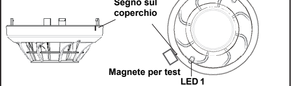
Figura 3: Posizione del magnete per il test
