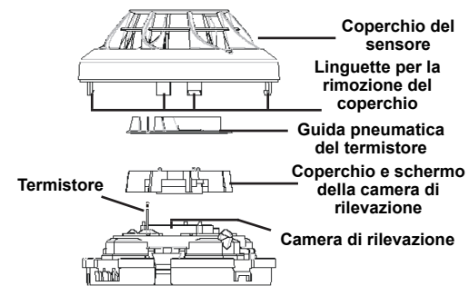
Figura 2: Pulizia del sensore
