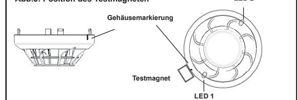
Abb.3: Position des Testmagneten
