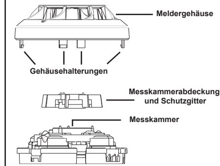
Abbildung 2: Reinigung des Melders
