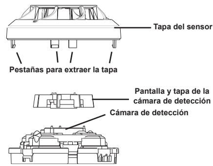
Figura 2: Limpieza del sensor
